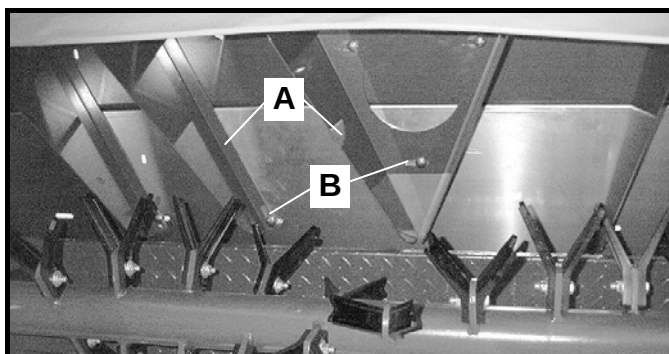
Abbildung 27: Leitbleche (Option)
