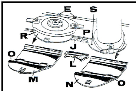
Abbildung 19: Messerschnellwechsel
