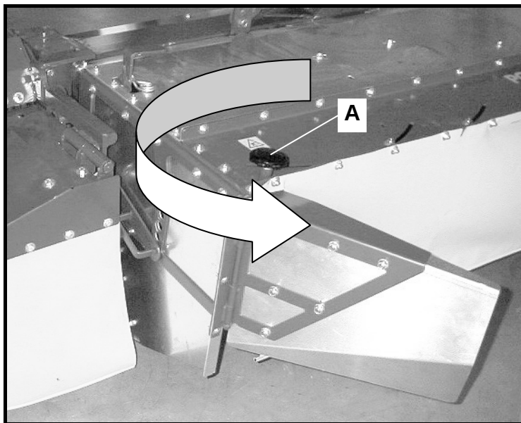
Abbildung 26: Schwadformer (Option)
