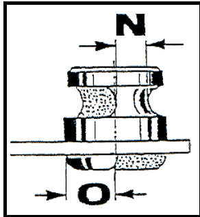
Abbildung 34: Verschleiß Messerzapfen
