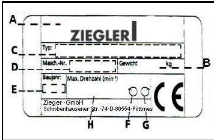
Abbildung 1: Maschinenschild
