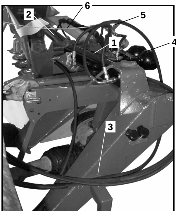
Abbildung 13: Hydraulik
