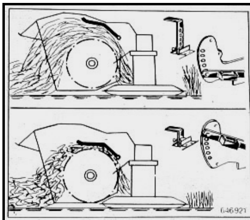
Abbildung 24: Label, Verstellung Knickzetter
