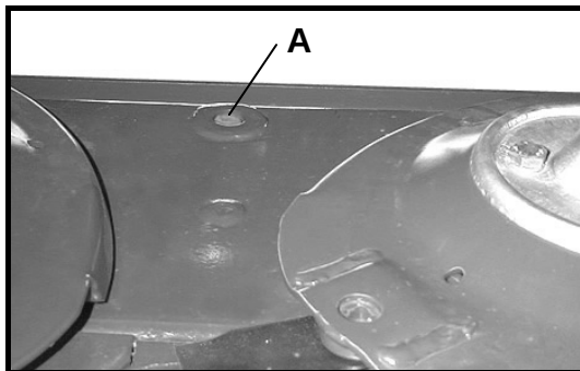
Abbildung 28: Einfüllöffnung Mähbalken
