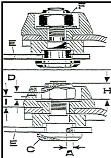
Abbildung 32: geschraubte Messerklinge
