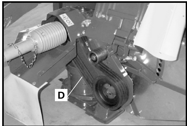
Abbildung 21: Knickzetterantrieb
