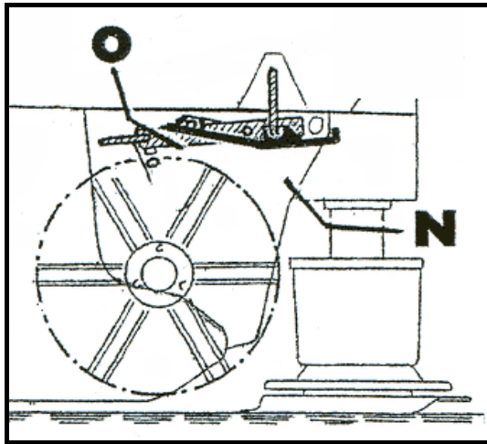
Abbildung 22: Prinzipskizze Knickzetter
