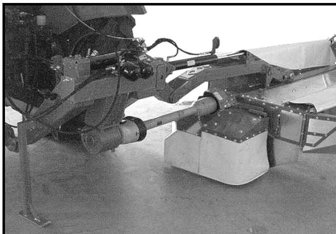
Abbildung 17: Winkelgetriebe
