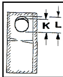
Abbildung 33: Verschleiß Messerklinge
