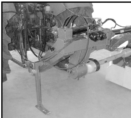
Abbildung 11: Gelenkwelle in Fahrtrichtung
