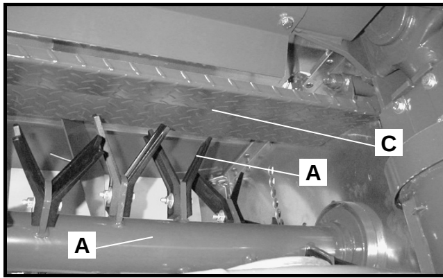
Abbildung 20: Knickzetter
