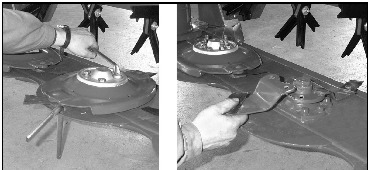
Abbildung 35: Messerhalterwechsel
