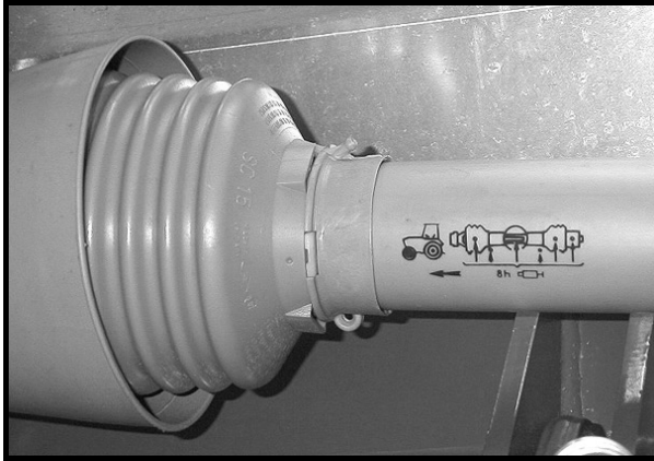
Abbildung 37: Wartung Gelenkwellen
