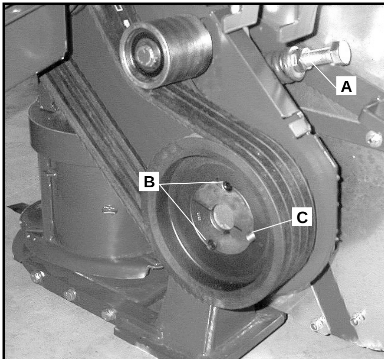
Abbildung 25: Keilriemenscheiben wechseln
