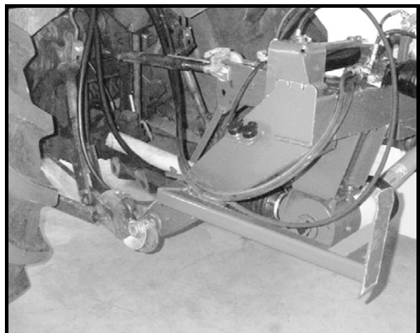
Abbildung 12: Geräteverriegelung
