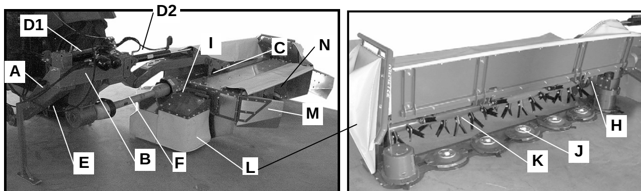
Abbildung 4: Gesamtansichten
