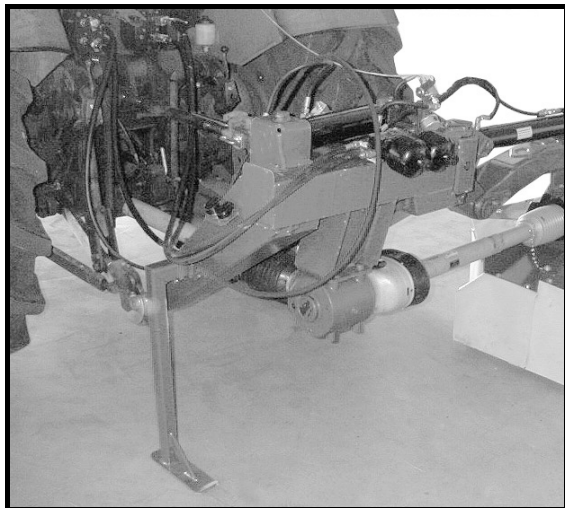
Abbildung 18: Abstellstütze
