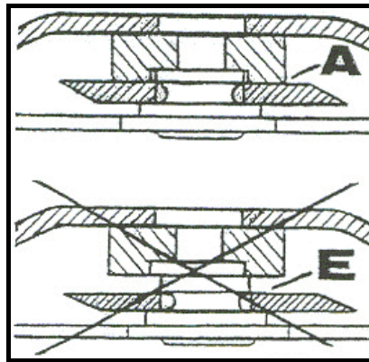
Abbildung 31: Position Messerhalterzapfen
