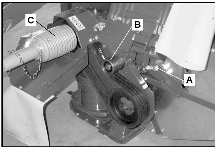
Abbildung 38: Knickzetterantrieb
